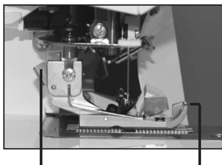
Рычаг освобождения лапки направителями прижимной лапки линии шва
