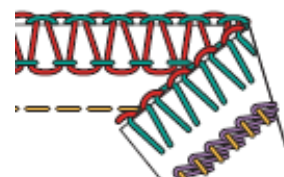
2-ниточная оверлочная строчка (RN) + Цепной стежок (LC)
