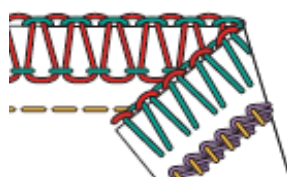
2-ниточная оверлочная строчка (LN) + Цепной стежок (LC)
