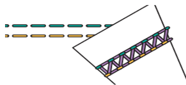
3-ниточный узкий расширительный шов (LC-CC)
