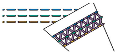
4-ниточный расширительный
