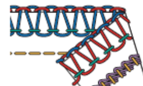
3-ниточная оверлочная строчка (RN) + Цепной стежок (LC)
