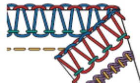
3-ниточная оверлочная строчка (LN) + Цепной стежок (LC)
