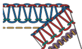
3-ниточная оверлочная строчка (LN) + Цепной стежок (CC)
