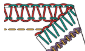
2-ниточная оверлочная строчка (RN) + Цепной стежок (CC)
