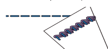
2-ниточная цепная строчка (RC)
