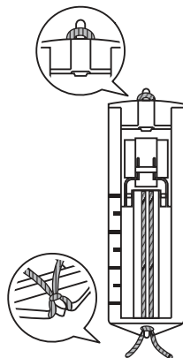
модель sew&go 1/3
