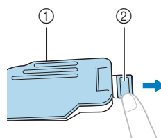
① Крышка челночного устройства ② Защелка
