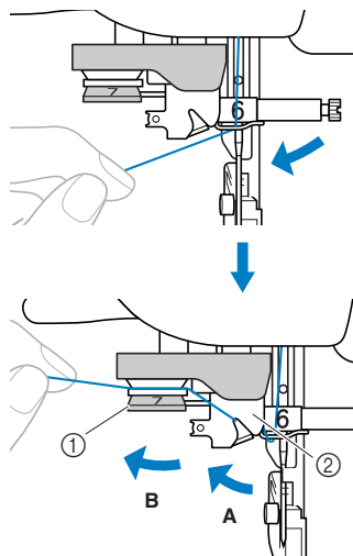
① Нитенаправляющий диск ② Нитенаправитель
