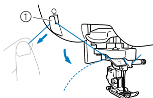
① Устройство для обрезки нити
